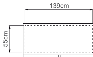
Vista superior
