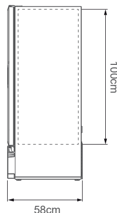
Vista lateral
